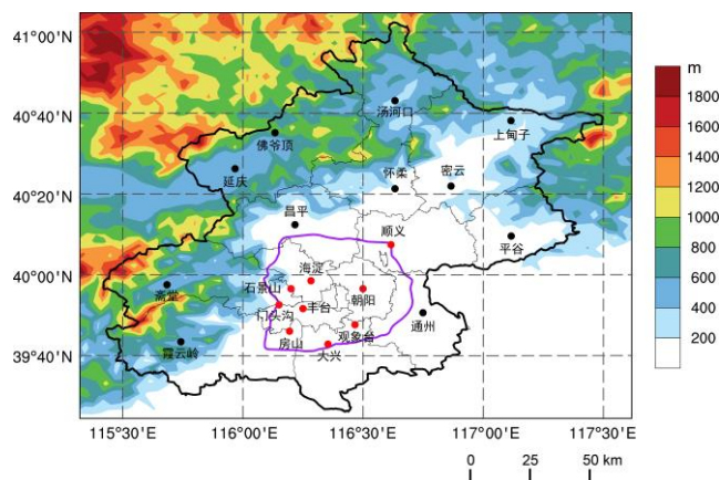
图 1 北京地区地形高度和自动气象站点分布
